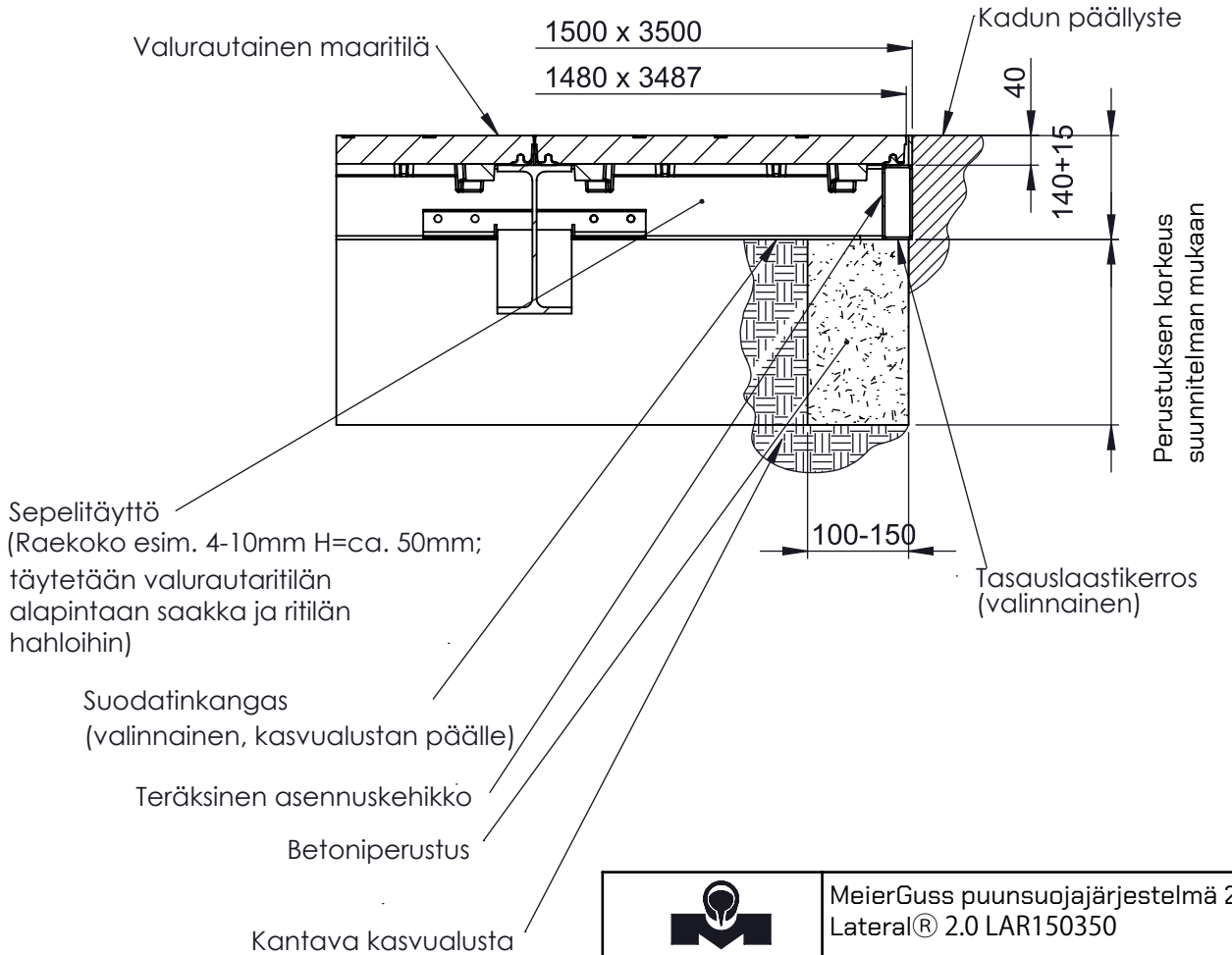
Maaritilän asennus, poikkileikkaus
