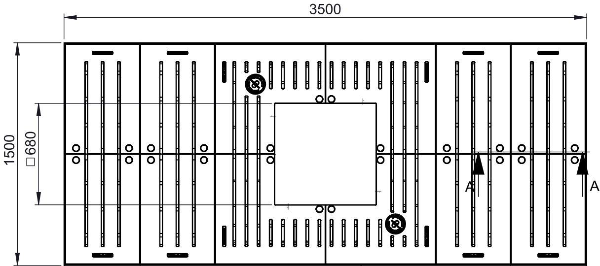
Yläkuvanto, kokoonpano ilman puun runkosuojaa
